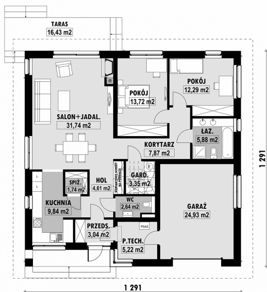
E-263-L PARTER
