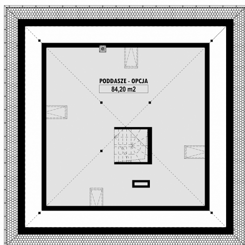
E-263-L PODDASZE
