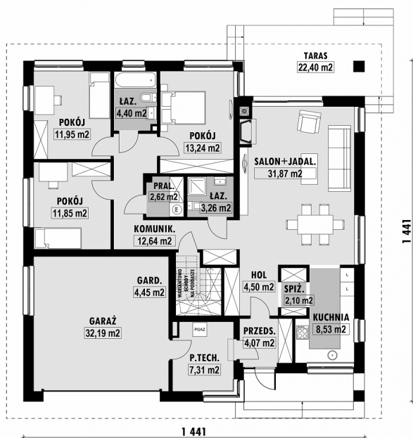
E-230a PARTER
