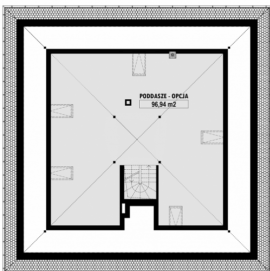
E-230a PODDASZE
