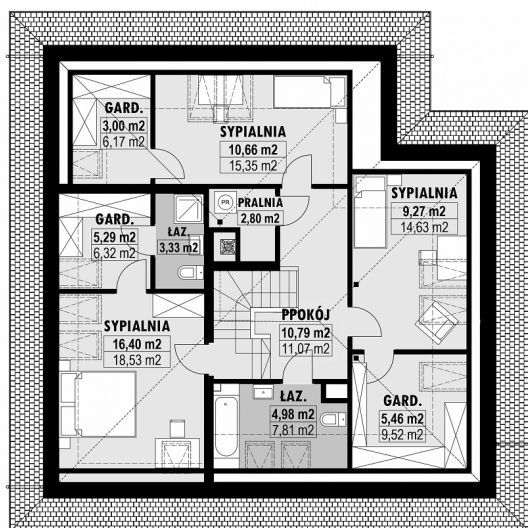
E-177 PODDASZE
