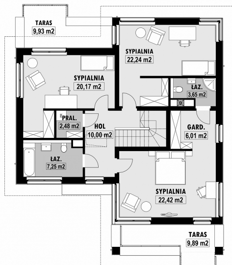
E-162-L PIĘTRO
