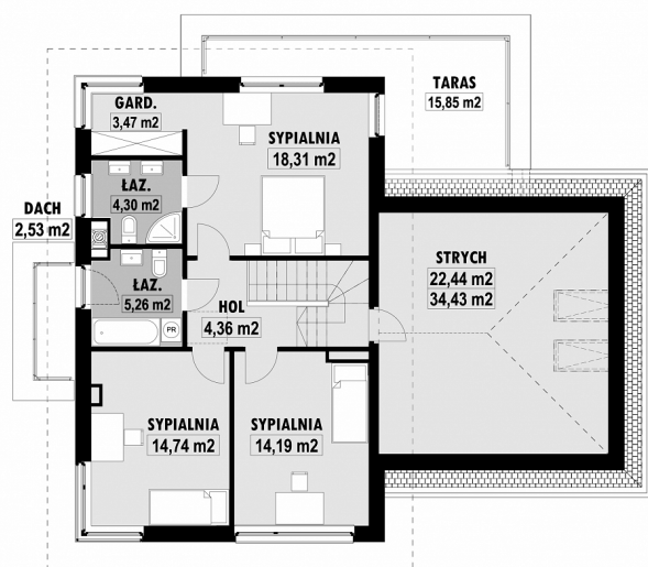
E-124-L PIĘTRO
