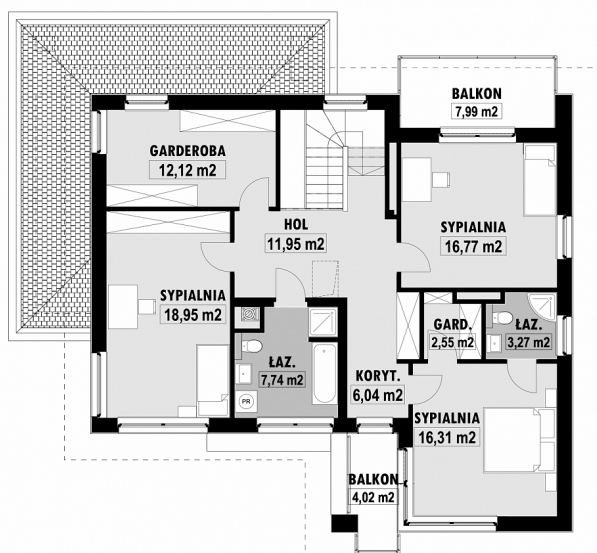
E-123-L PIĘTRO
